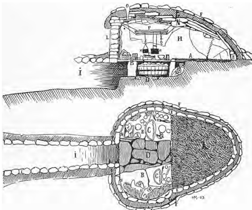
Snit gennem et polar-øskimoisk hus. A, sovebriks. B, sidebriks. C, lamper. D, gulv. E og F, stenmur. G, græstørv. H, rum over briksen. I, husgang. J, kasse med kød. K, kvindekniv. L, tarmskinsrude. M, gryder. O, ventil. P, tørrehække. R, rum under briksen. (Tegning af Harald Moltke).
