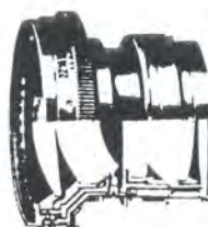
Sonnar 1:2 f=5 cm (versenkbare Fassung)
