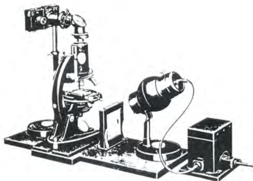
Mikroskopopstilling med prismeforsats.
