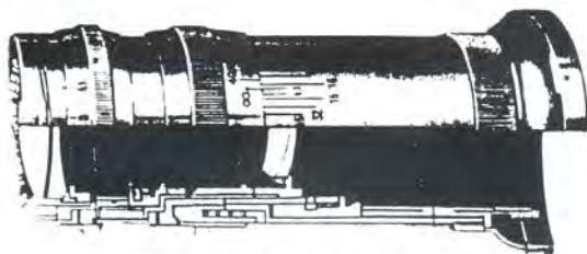
Tele-Tessar K 1:6,3 f=18 cm
