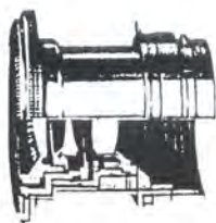
Tessar 1:3,5 f=5 cm
